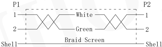
Wiring Table
